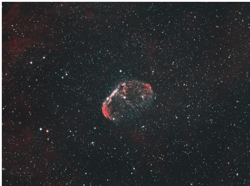
「NGC6888 三日月星雲」
