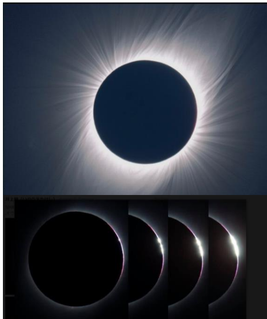
南米チリでバッチリみえた皆既日食 2019年7月2日 チリ・コキンボ州 とアタカマ州の州境で撮影。
