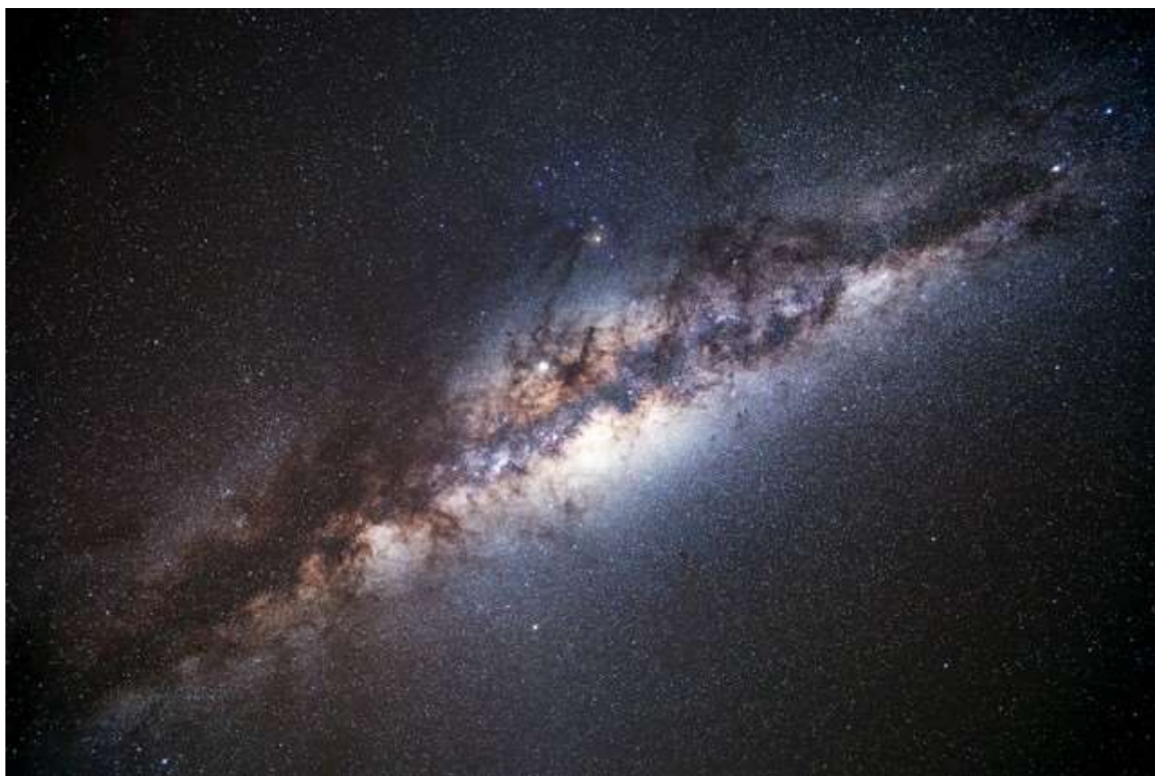
南天・銀河中心(@Australia Springhills Farm)
