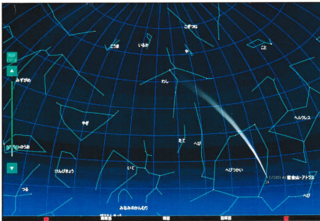
2024年10月20日 19時20分の彗星予報
